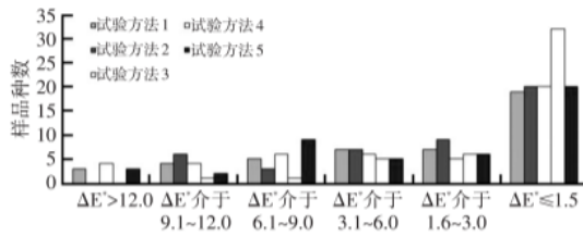
图 4 样板经 1200 h 氙灯试验的颜色变化分布
