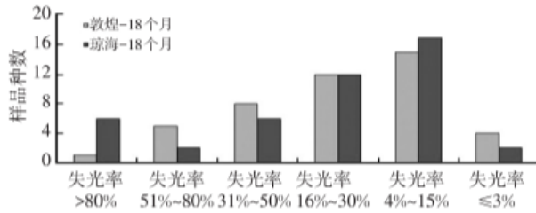
图 1 样板户外曝晒 18 个月的失光率分布
