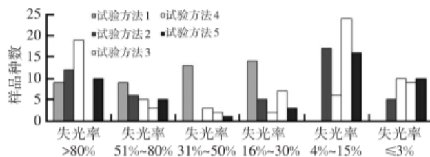
图 3 样板经 1200 h 氙灯试验的失光率分布
