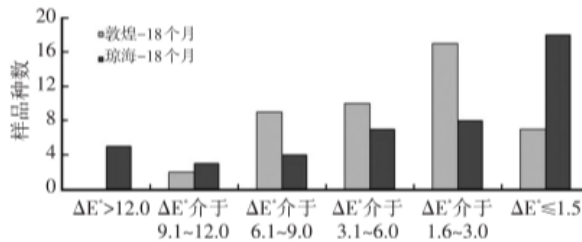
图 2 样板户外曝晒 18 个月的颜色变化分布
